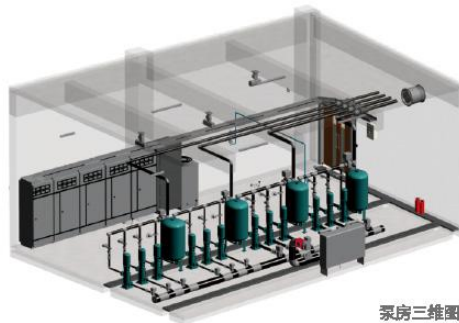
泵房三维图
